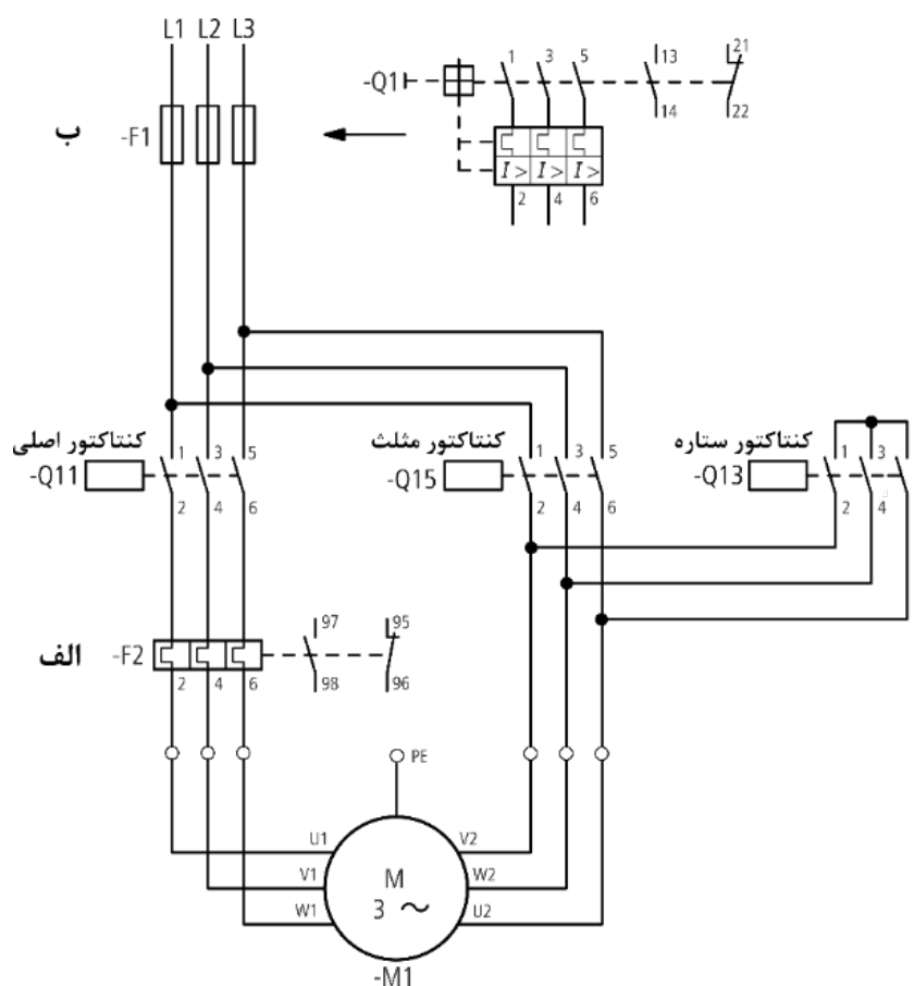
شکل ۶-۶۵- مدارهای راه اندازی موتور الکتریکی به روش ستاره-مثلث
