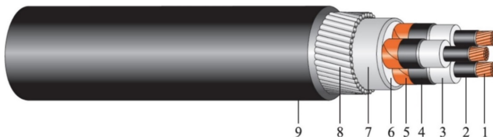
شکل ۳-۱۵- اجزا مختلف یک نمونه کابل فشار متوسط تک رشته‌ای N2XSRY
