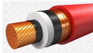
شکل ۳-۳- کابل تک رشته‌ای
