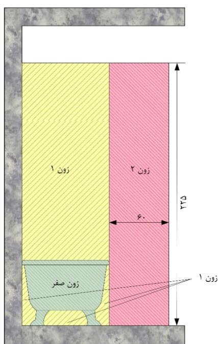
شکل ۴-۶- ابعاد زون‌ها: دید از کنار وان
