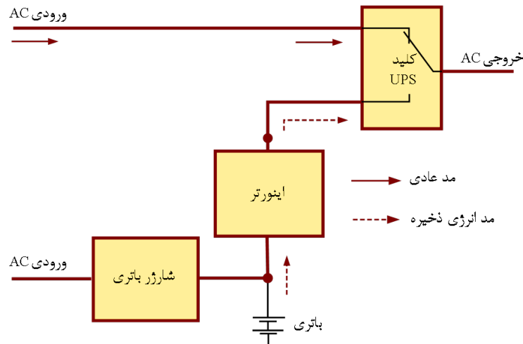
شکل ۱۰-۱- توپولوژی آماده به کار
