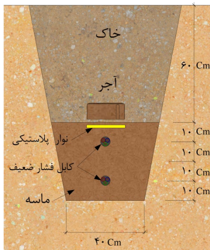
شکل ۲-۷- جزئیات کانال خاکی تیپ، برای نصب کابل فشار ضعیف در دو ردیف افقی
