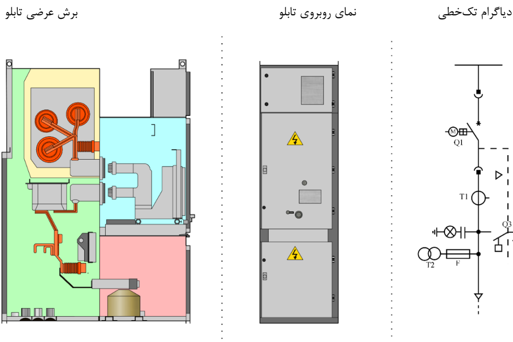
شکل ۷-۱۷- الف: تابلوی فشار متوسط در سطح اولیه با کلید قدرت کشویی، CT، PT، فیوز مربوط، کلید زمین و مقسم ولتاژ خازنی که می‌تواند نقش تابلو ورودی یا خروجی را ایفا کند.
