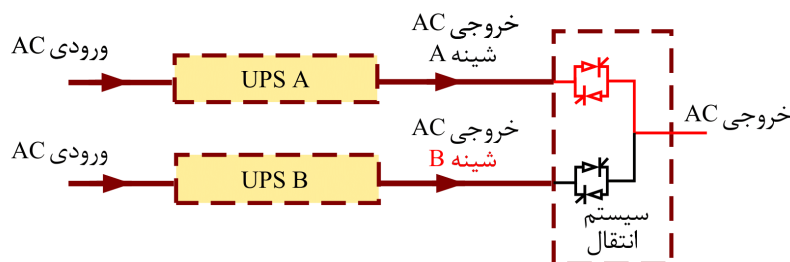
شکل ۱۰-۷- UPS دو خروجی جایگزین آماده به کار
