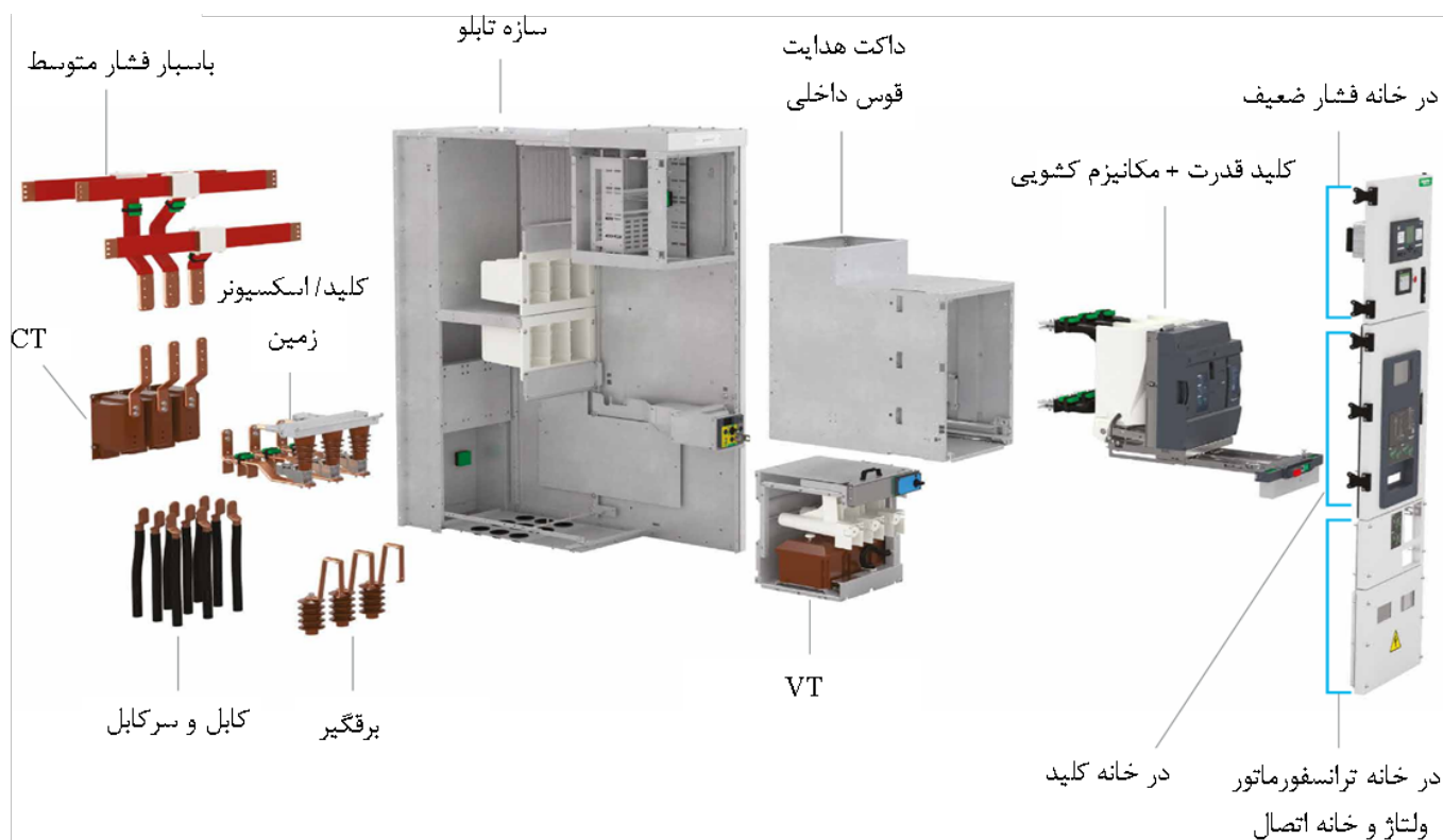
شکل ۷-۱۴- اجزا تابلو فشار متوسط نمونه
