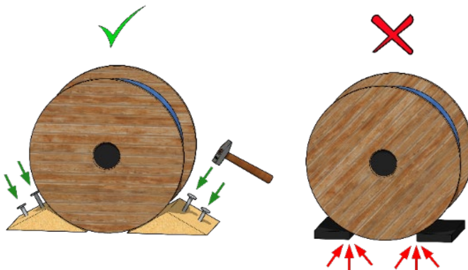
شکل ۳-۲۱- مهار کردن قرقره کابل‌ها با گوه
