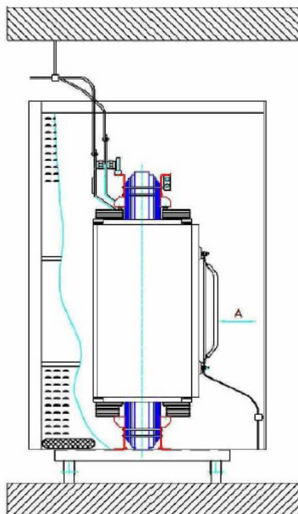
آرایش سه: ترمینال‌های فشار ضعیف از بالا و ترمینال‌ها و کابل‌های فشار قوی از پایین. شکل ۸-۲۷- راهنمای انتخاب آرایش اتصالات ترانسفورماتورهای خشک در محفظه فلزی (ادامه)
