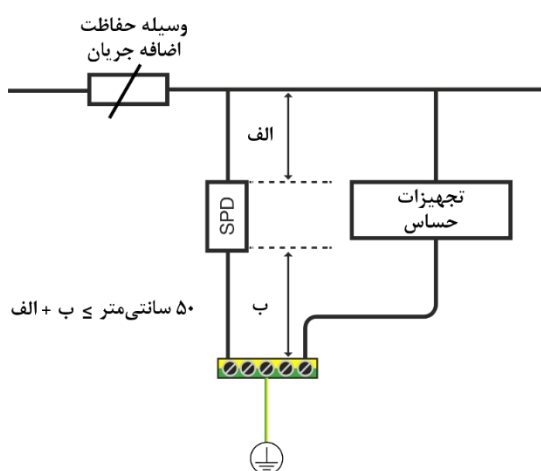
شکل ۶-۵۷ - سیم‌کشی صحیح SPD
