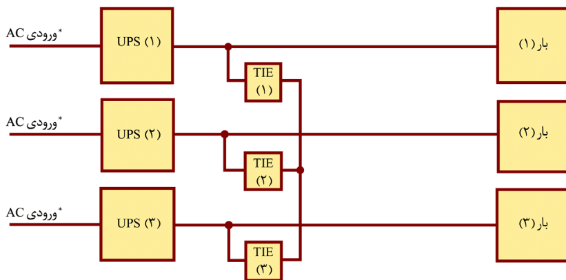
شکل ۱۰-۲۰- کلید رابط در کاربردهای دومسیره
