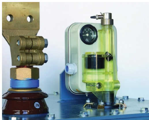
شکل ۸-۱۷- رله چندکاره ترانسفورماتور هرمتیک کنگره‌ای
