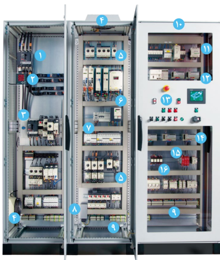
شکل ۶-۳- کنسول کنترل یا تابلو برق بیانویی
