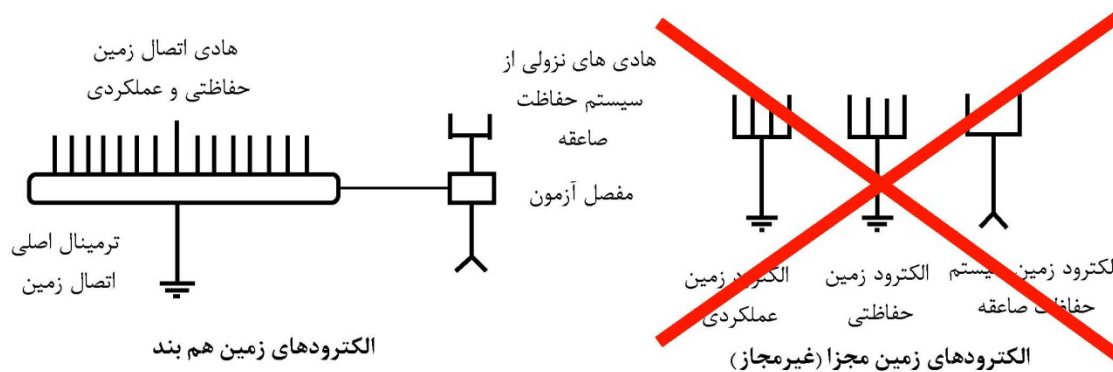
شکل ۱۴-۶- هم‌بندی الکترودهای زمین
